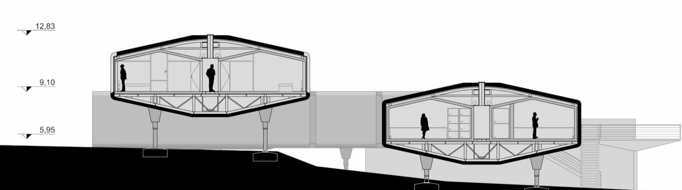
CORTE DD' 1/250
