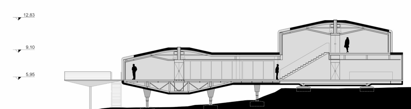
CORTE CC' 1/250
