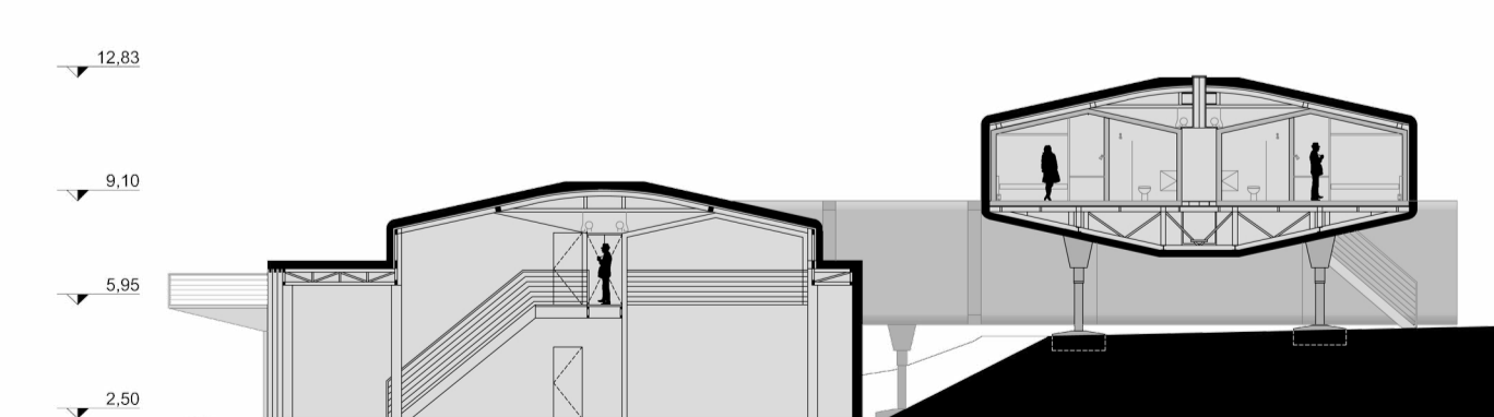
CORTE EE' 1/250
